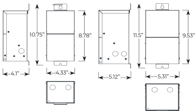
VLT600150A
